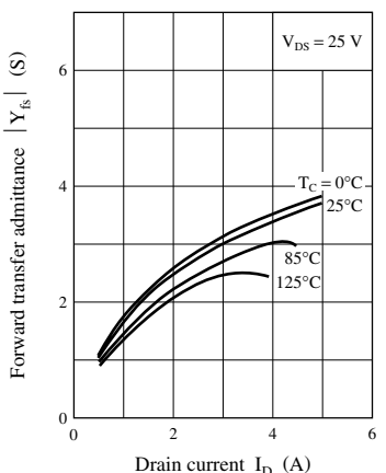
|Y_{fs}| - I_D
