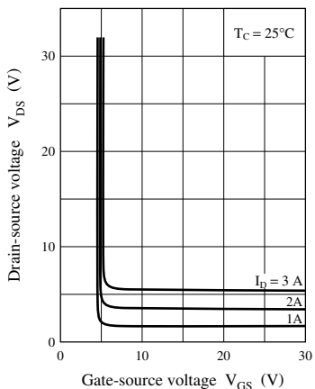
V_{DS} - V_{GS}
