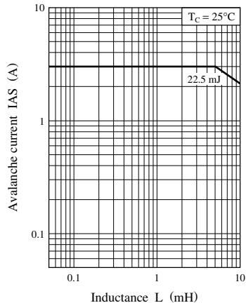
IAS — L
