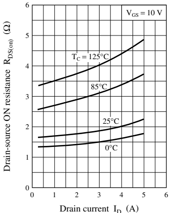
R_{DS(on)} - I_D
