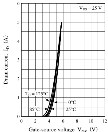
I_D - V_{GS}
